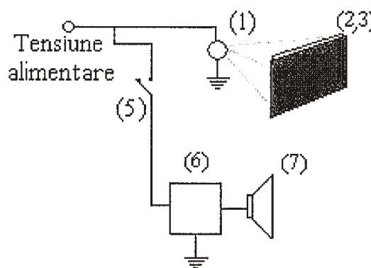
circuitul audio
