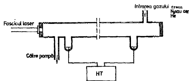
Schema de principiu a unui laser cu freon
